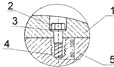
Szczegół A
