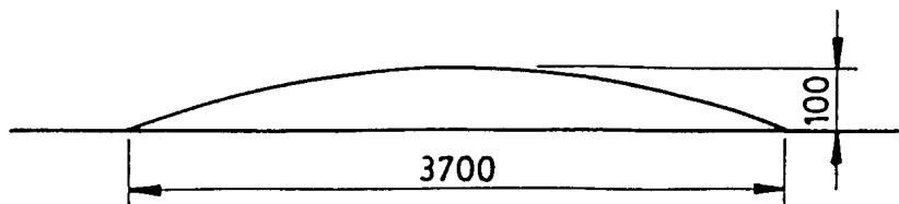
a. Próg listwowy typu 1
