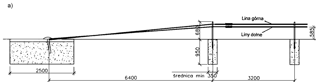
Rys. 6. Przykłady ukośnego odcinka początkowego bariery liniowej a) Bariera trzylinowa, b) Bariera czterolinowa
