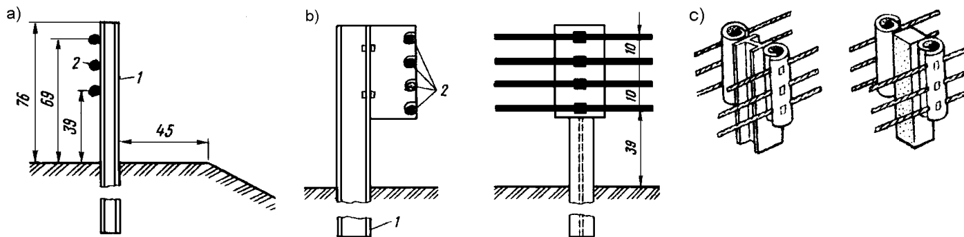
Rys. 3. Przykłady umocowienia lin do słupków a) Bariera trzylinowa, b) Bariera czterolinowa, c) Bariera trzylinowa dwustronna na słupku dwuteowym i prostokątnym, 1 – słupek, 2 – lina
