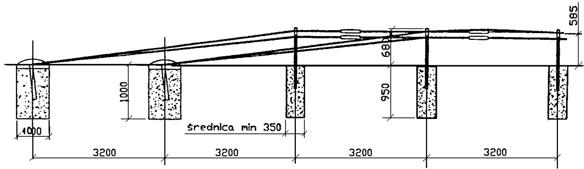
Rys. 7. Przykłady lin stalowych stosowanych w barierach linowych
