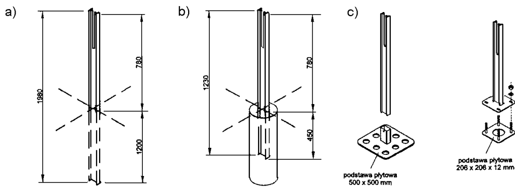
Rys. 5. Sposoby osadzenia w gruncie i przymocowania słupków barier liniowych a) Słupek zagłębiony w gruncie, b) Słupek osadzony w fundamencie betonowym, c) Słupki z metalową podstawą płytową do przymocowania na obiekcie mostowym
